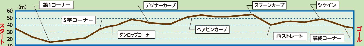
鈴鹿サーキット国際レーシングコース高低差図(フルコース1周5.807km)
